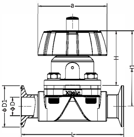
XBI-2G81FI6R基本尺寸 Dimension of XBI-2G81FI6R 单位Unit:mm
